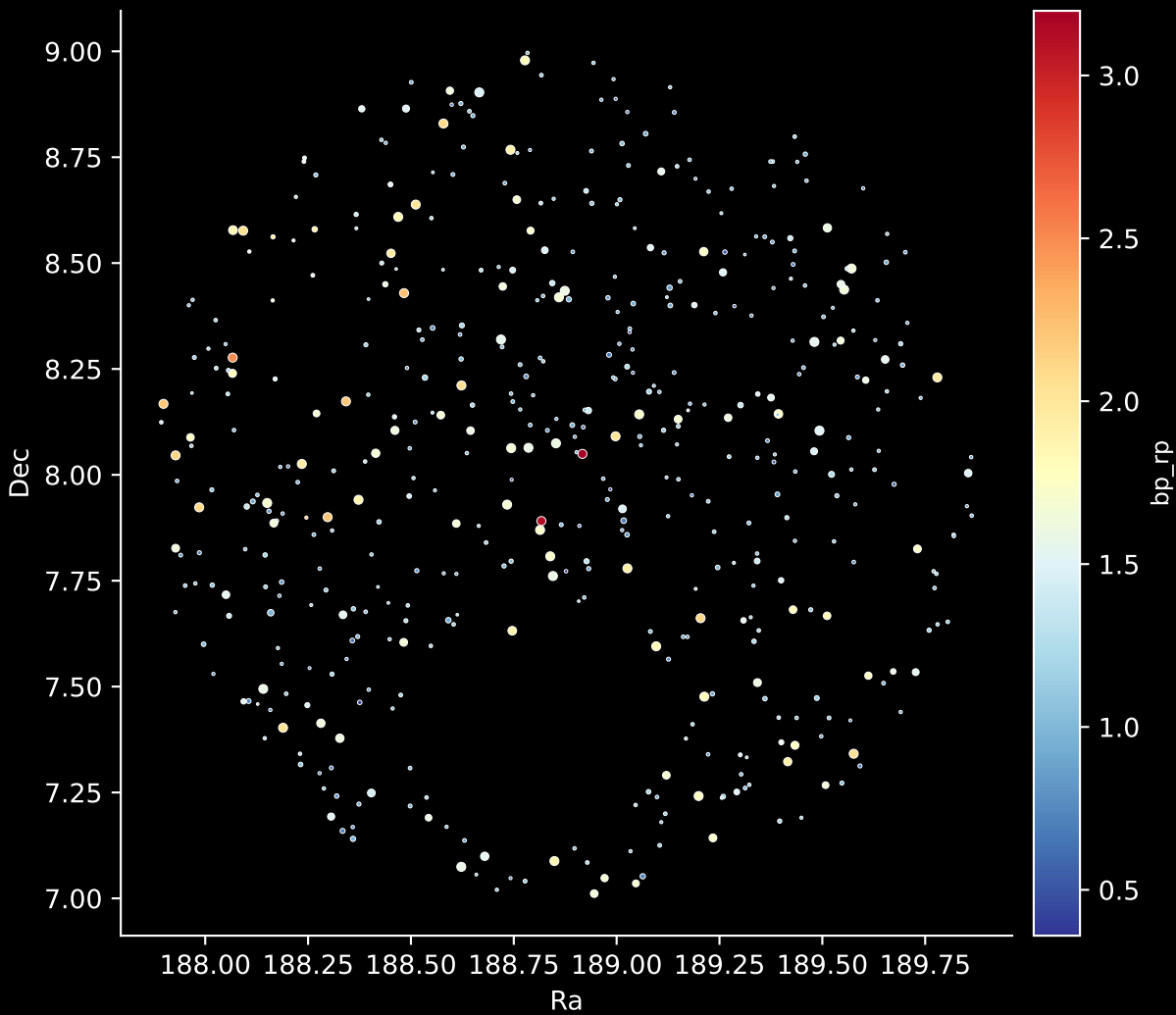
GALAH DR4 Field: [9467] Stars: 495
