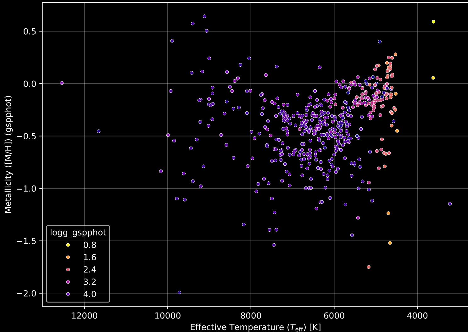
GALAH DR4 Field: [9467] Stellar Population Parameters (n= 495)
