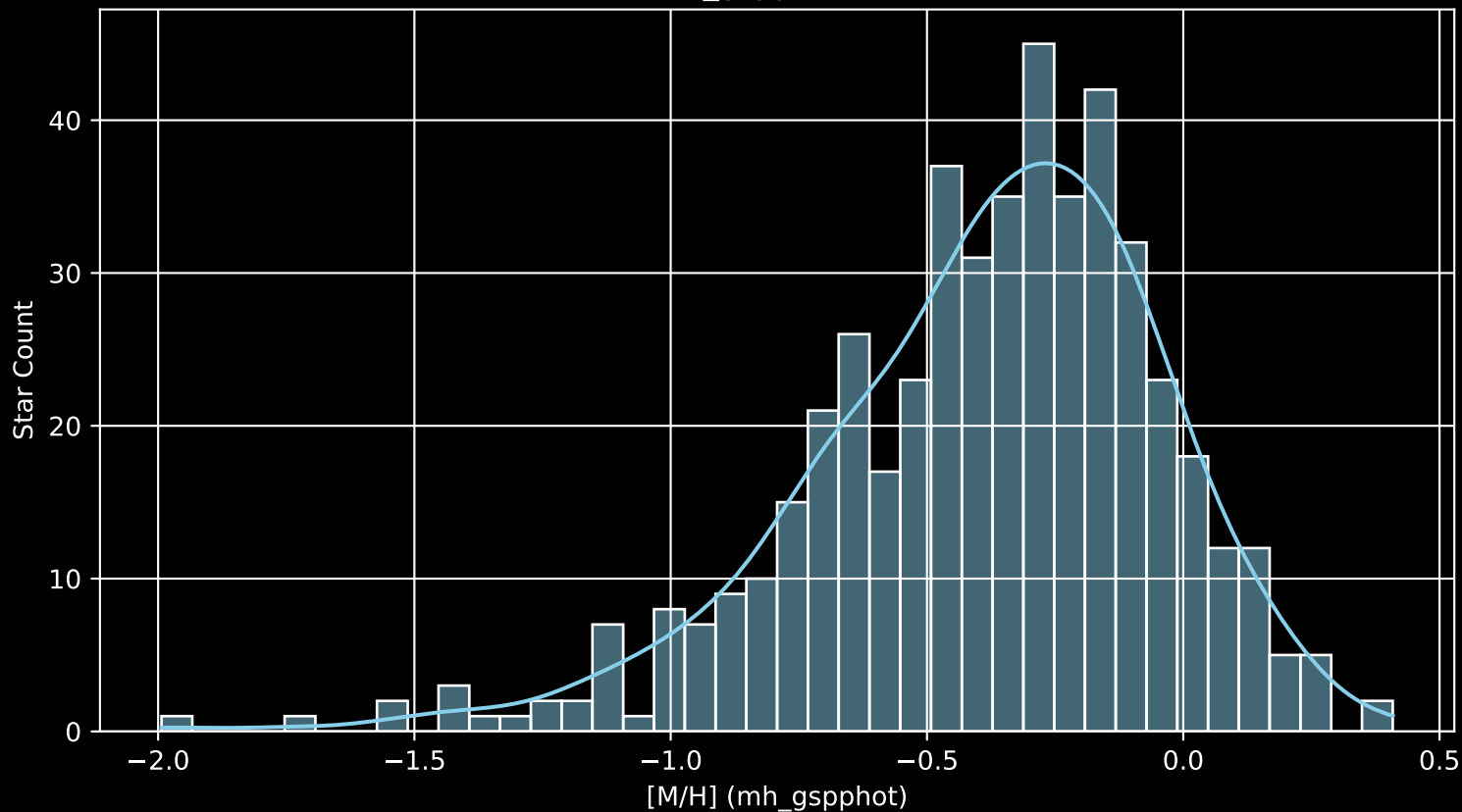
GALAH DR4 Field: [9467] [M/H] (mh_gspphot) (n= 491)
